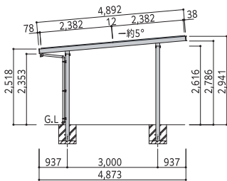
側面図 [1台用]
